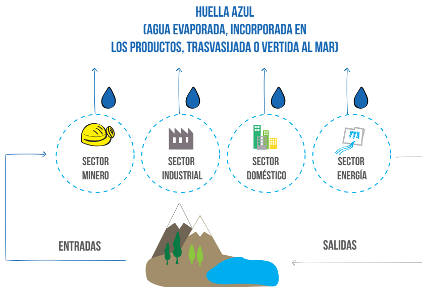
Figura 6: Huella Hídrica del sector agrícola.
