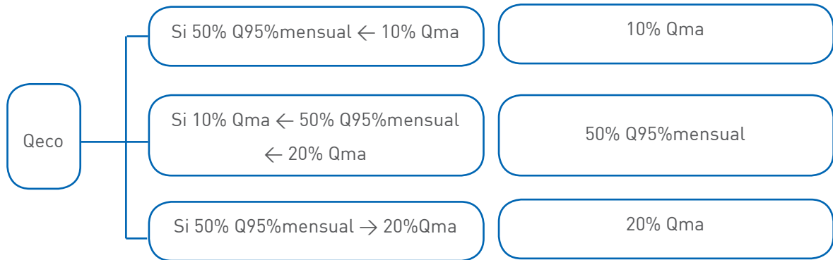
Figura 10: Criterios utilizados para determinar el caudal ecológico mínimo. Fuente: Elaboración propia.
