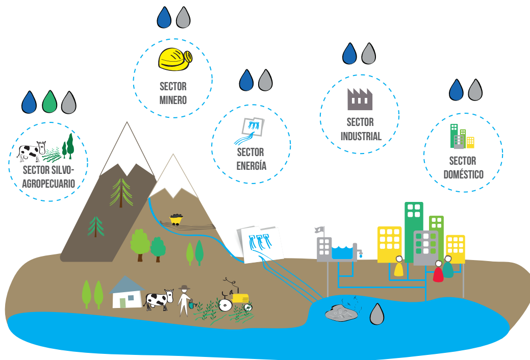
Figura 4: Medición de la Huella Hídrica en cuenca.
