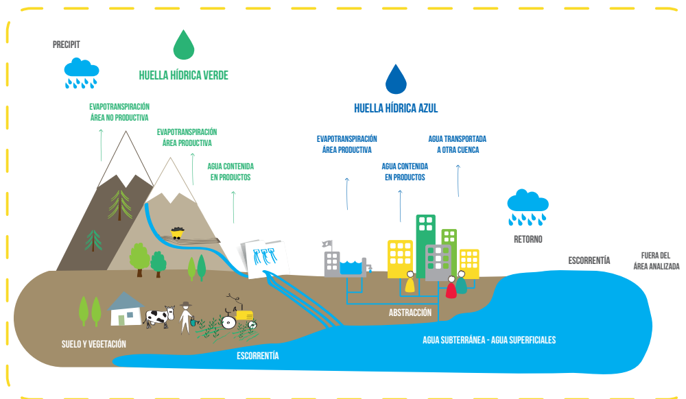
Figura 1: Relación entre las huellas hídricas azul y verde y el balance hídrico de la cuenca.
