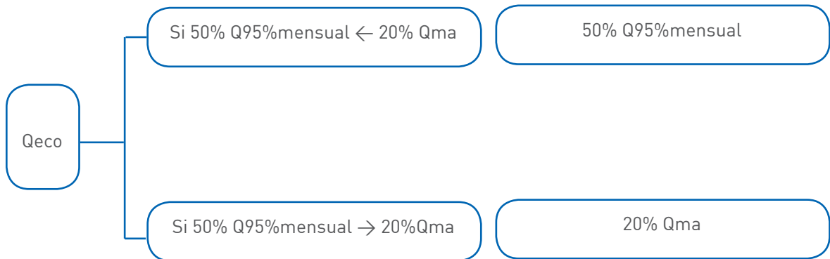
Figura 11: Restricciones para determinar el caudal ecológico mínimo. Fuente: Elaboración propia.
