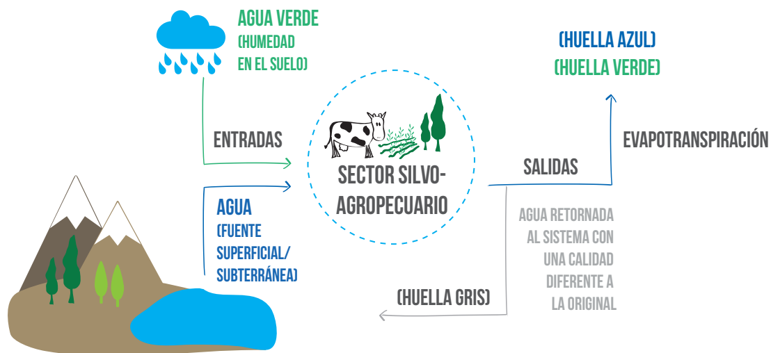
Figura 5: Huella Hídrica del sector agrícola. Fuente: Elaboración propia.
