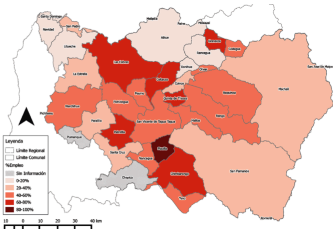
Figura 8: Porcentaje de empleo que está relacionado con el sector silvo-agropecuario, a nivel comunal, en la cuenca del Río Rapel.
