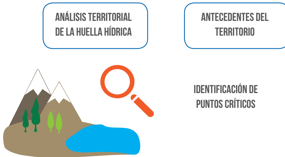
Figura 7: Análisis de sustentabilidad de la Huella Hídrica. Elaboración propia Fuente: Elaboración propia.
