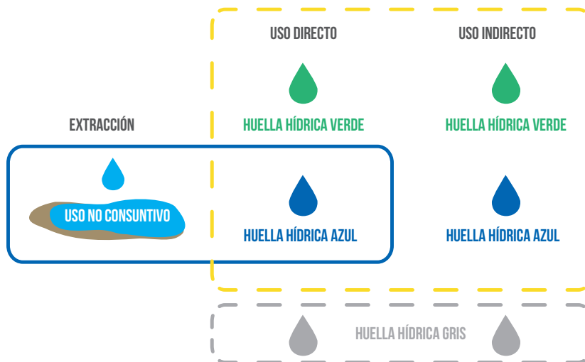
Figura 2: Representación esquemática de los componentes de la Huella Hídrica Fuente: Elaboración propia en base a Hoekstra, et al. (2011).
